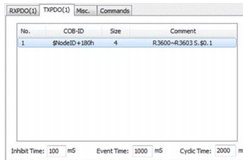
图 40: 移除 TXPDO
