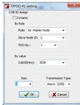
图 53: TXPDO 设定
