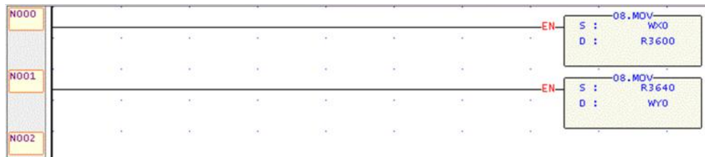
图 63:FBs-24M C 及 FBs-20M C 的 Ladder 程序
