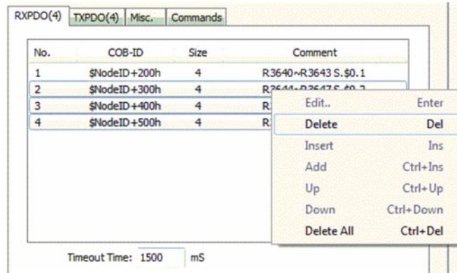
图 37: 删除 RXPDO
