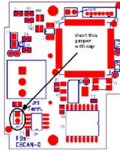
图 4:Temp jumper位置
