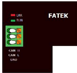
图 1: CBCAN 上视图
