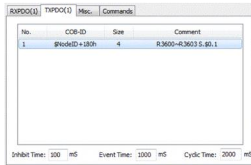
图 52: 移除 TXPDO
