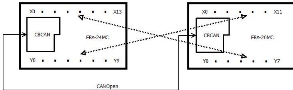
图 56: FBs-24M C 和 FBs-20M C 点对点通讯
