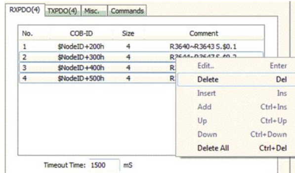
图 49: 移除 RxPDO
