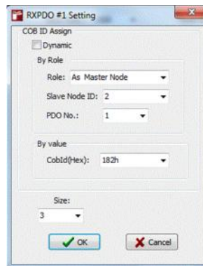
图 51: 此范例中的 RXPDO1 设定
